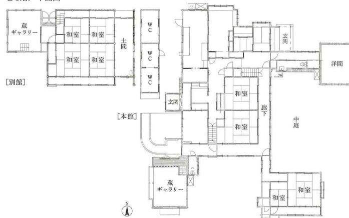
◎1階/平面図
