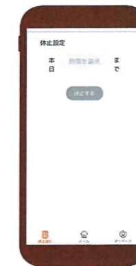
休止設定
