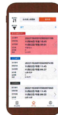
注文管理
