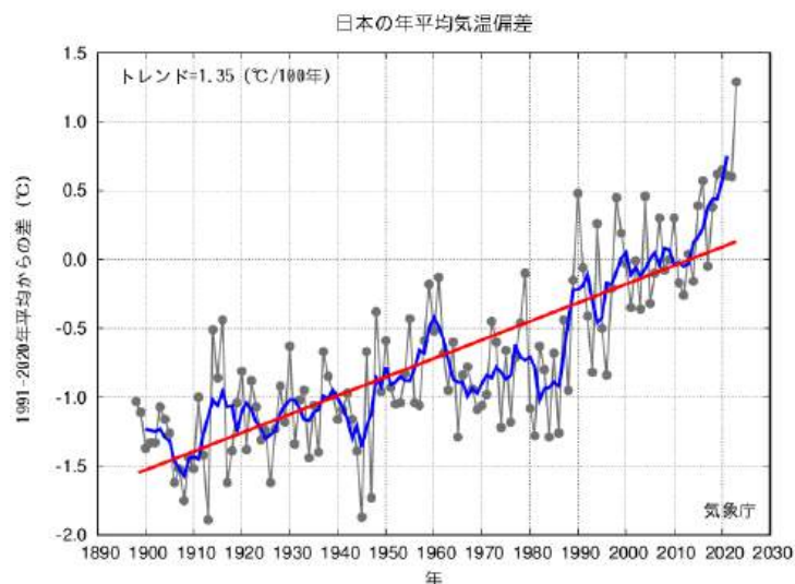
日本の年平均気温偏差の経年変化（1898～2023年）
