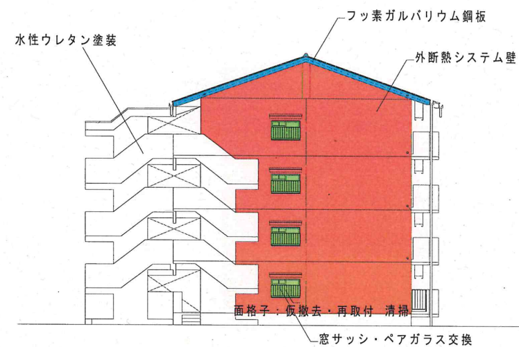
南立面図 S=1/200
