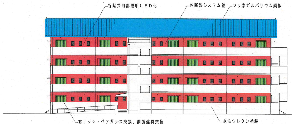
西立面図 S=1/200
