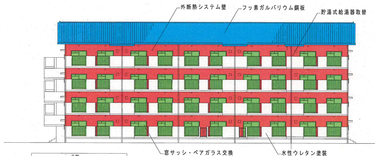
東立面図 S=1/200
