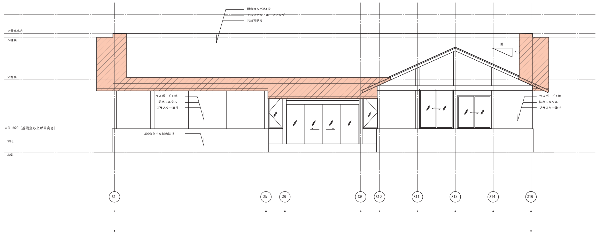
東側立面図
