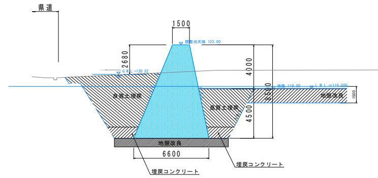
A-A' 断面図 重力式コンクリート擁壁部
