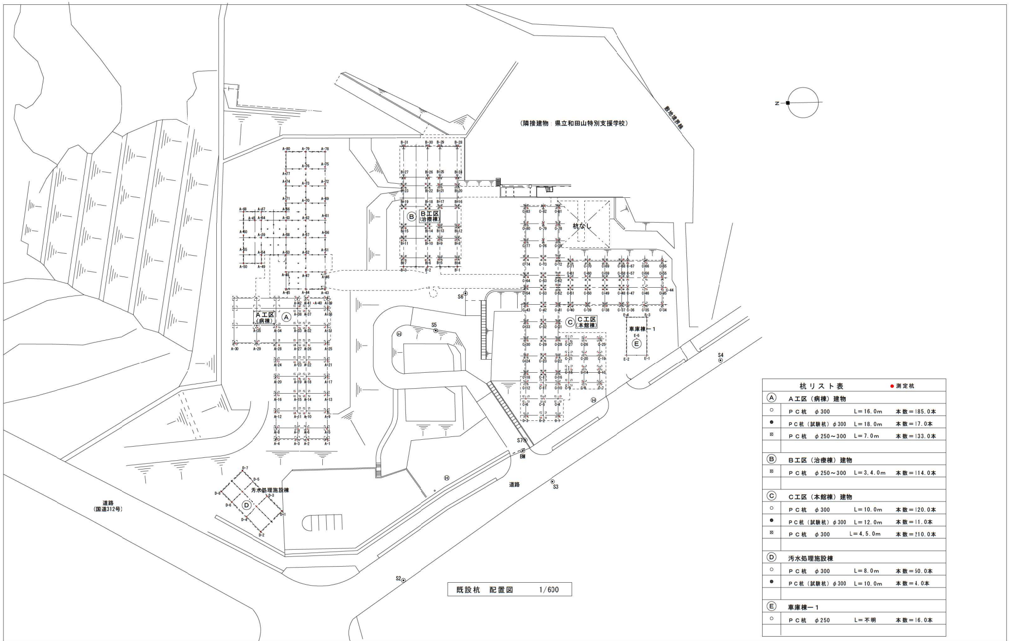
旧公立朝来和田山医療センター跡地 地中杭位置図
